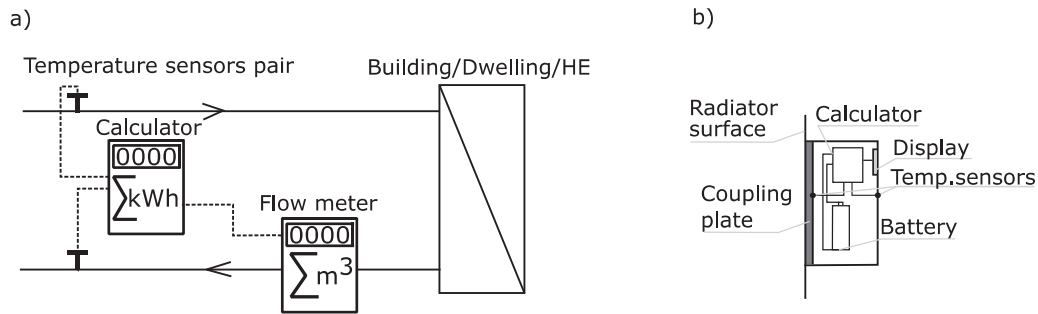
Fig. 4. a) DHM and b) HCA functioning scheme.
